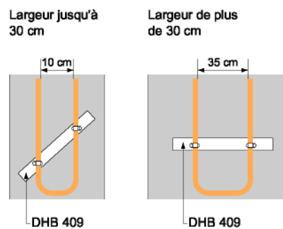
Montage dans des sheds ou toits plats
