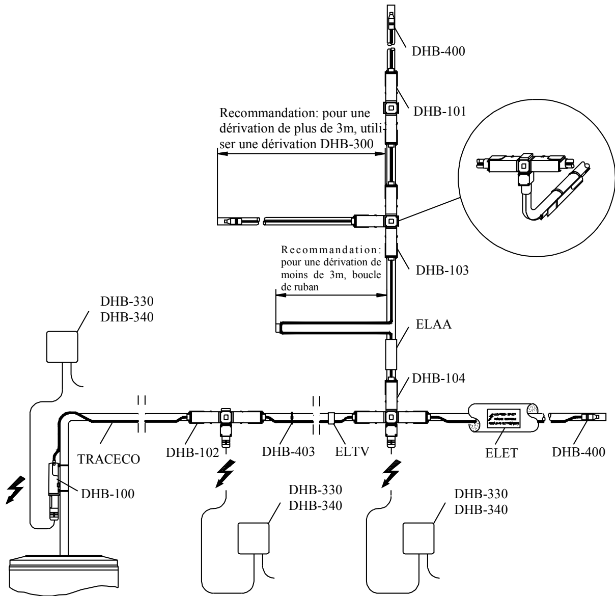
Alimentation Variante 1 Au début/A la fin du ruban chauffant
